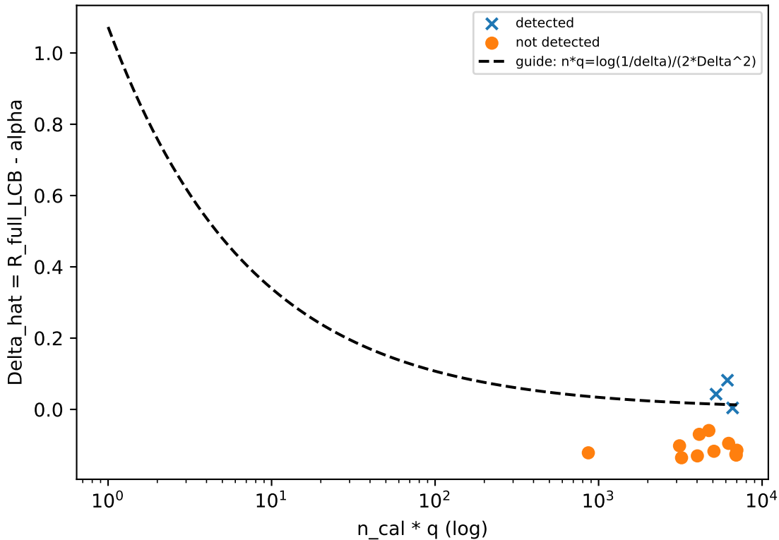
F4 detection -- tabular-MiniBooNE[margin]
